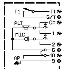
Rys. 2 oznaczenia zacisków unifonu
