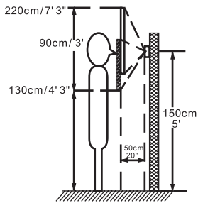
WIDOK BOCZNY
